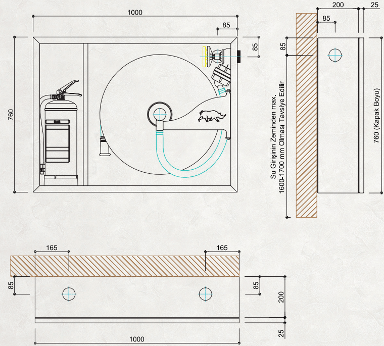
SIVAÜSTÜ TİP
